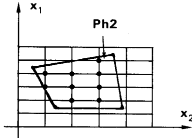
Figure 4. — Schéma de discrétisation d'un polyèdre.
