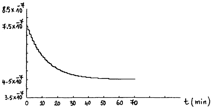
Figure 3. — La concentration de la protéine kinase (C) en fonction du temps donnée par le modèle.
